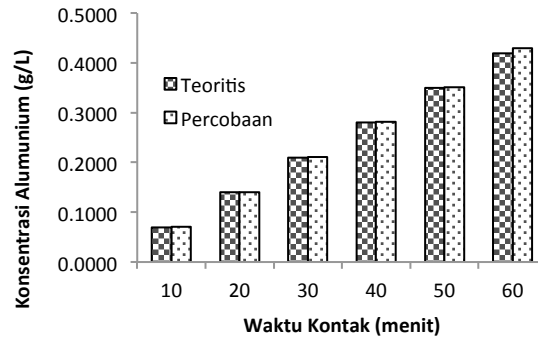
Gambar 5. Perbandingan konsentrasi alumunium teoritis dan percobaan yang terlepas selama proses elektrokoagulasi pada kerapatan arus 104 A/m 2
