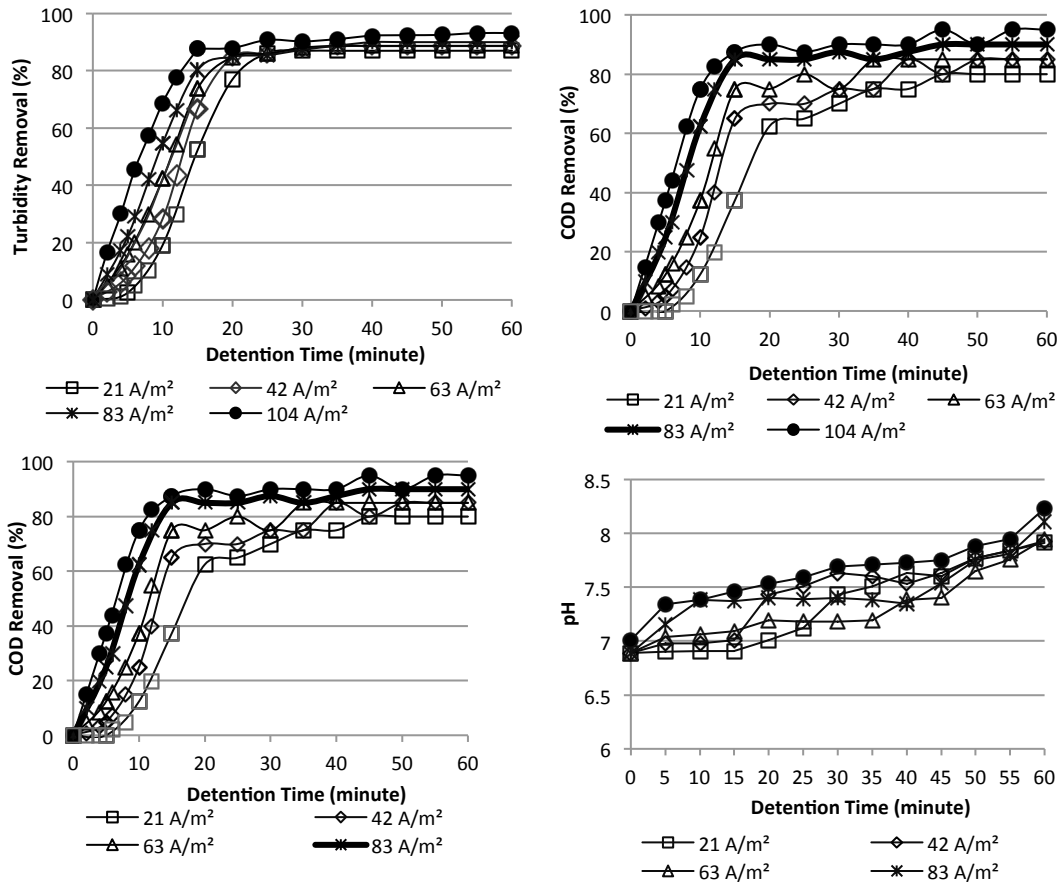
Gambar 2. Efisiensi penyisihan pada variasi kerapatan arus dan waktu detensi
