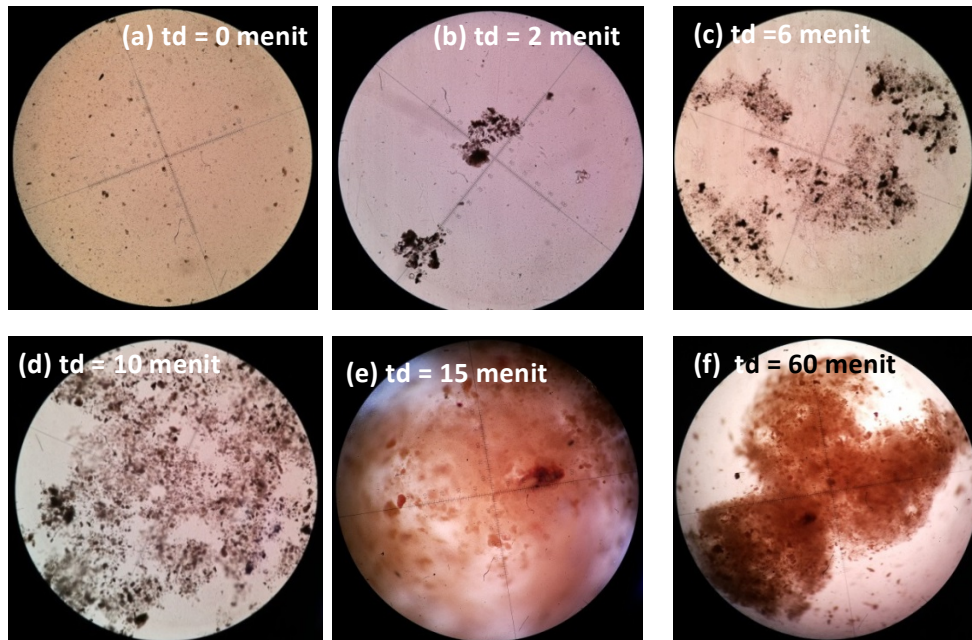
Gambar 4. Bentuk dan ukuran flok pada kerapatan arus 104 \text{ A/m}^2 (a-e) Pembesaran 10 x, (h) Pembesaran 4 x
